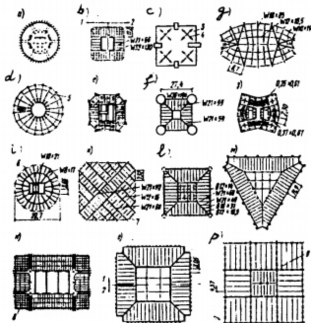
Hình VII.3. Những kết cấu sàn thông dụng
