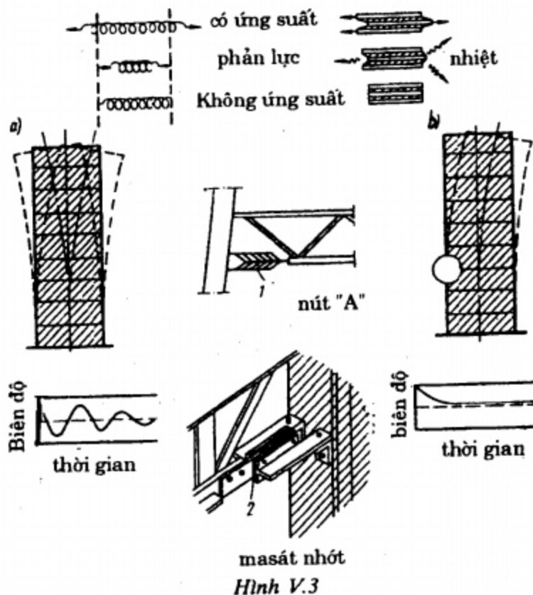
a- Không có hệ thống giảm chấn cơ học (chỉ có bộ hãm bên trong) ; b- Có bộ hãm. 1- Sơ đồ bộ giảm chấn ; 2- Dệm đàn hồi dẻo.
