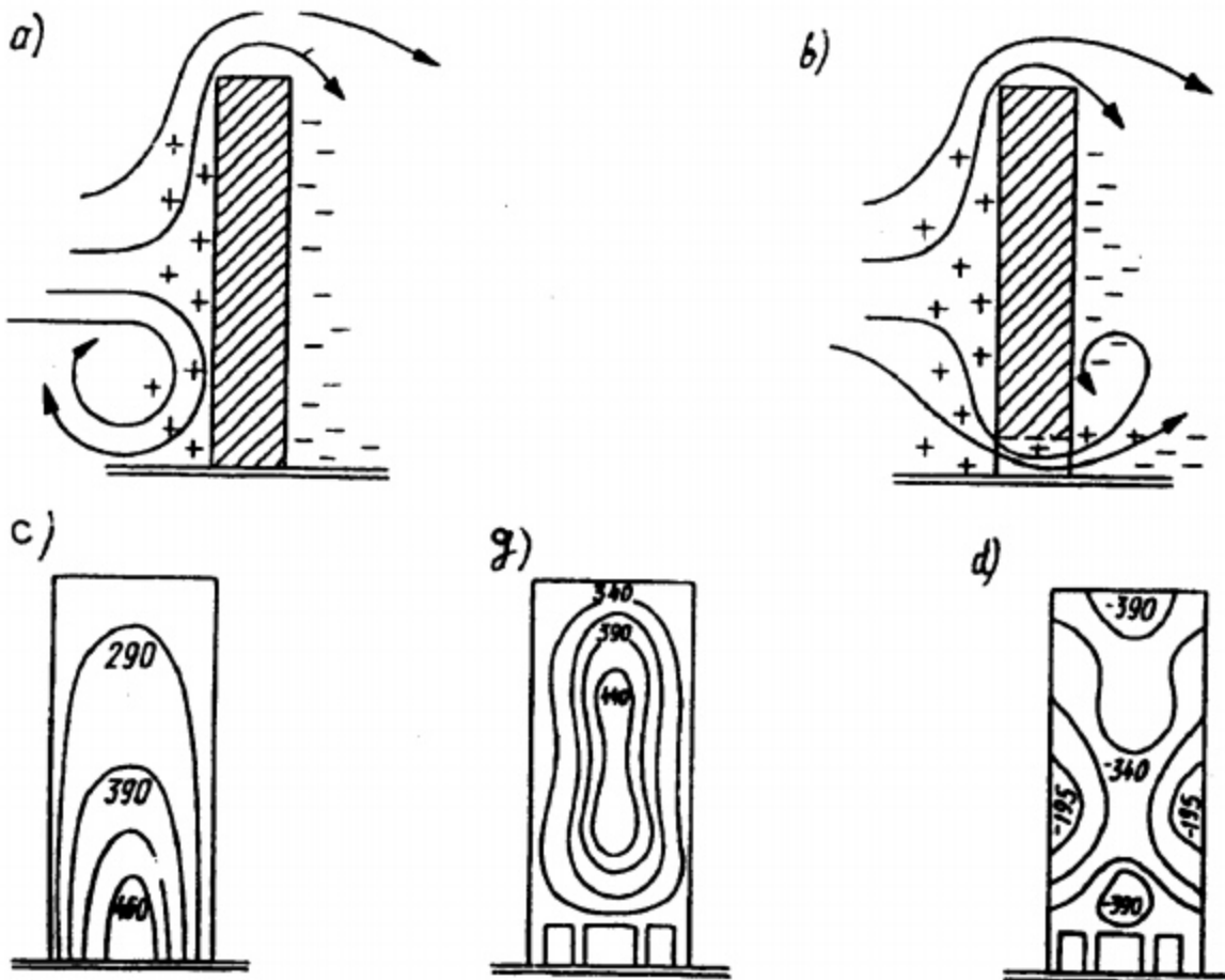
Hình 1.8- Đường đẳng áp lực gió theo kết quả quan sát ở trung tâm MIT [I. 15]
