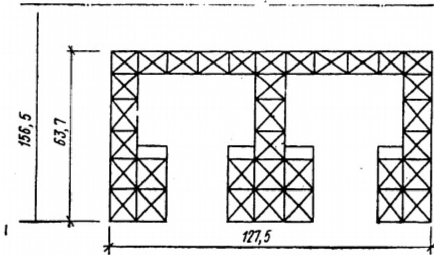
Hình IX.19- Mặt bằng ngôi nhà VAB
