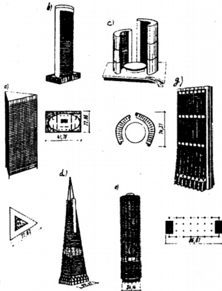
Hình V.1- Hình dạng hợp lý của ngôi nhà
