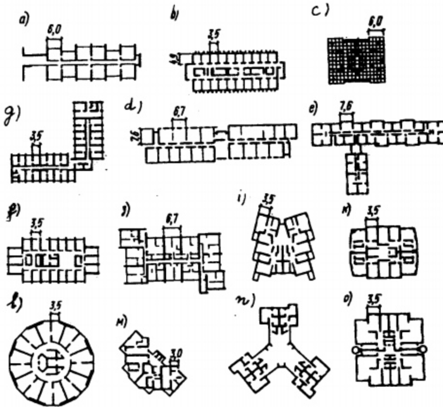
Hình IV.1. Sơ đồ các nhà có tường chịu lực phẳng
