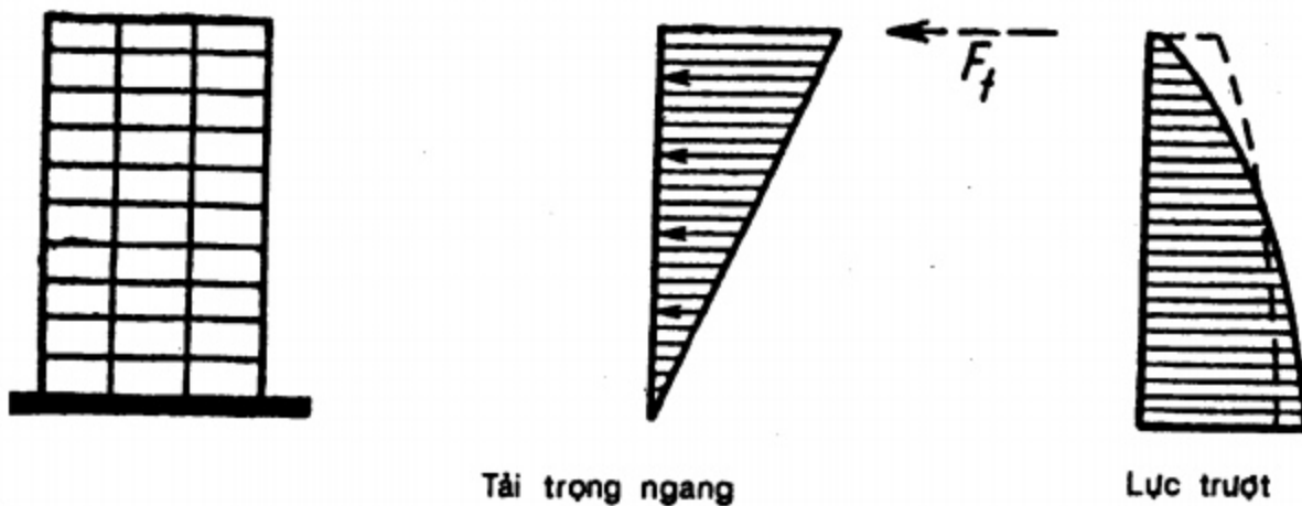
Hình 1.20- Sự phân bố của tải trọng động đất theo phương ngang theo yêu cầu của Tiêu chuẩn xây dựng Thống nhất
