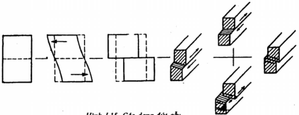
Hình 1.15. Các dạng đứt gãy
