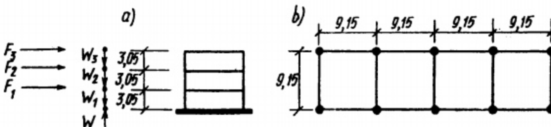
Hình I.23 a- Mặt cắt ; b- Mặt bằng
