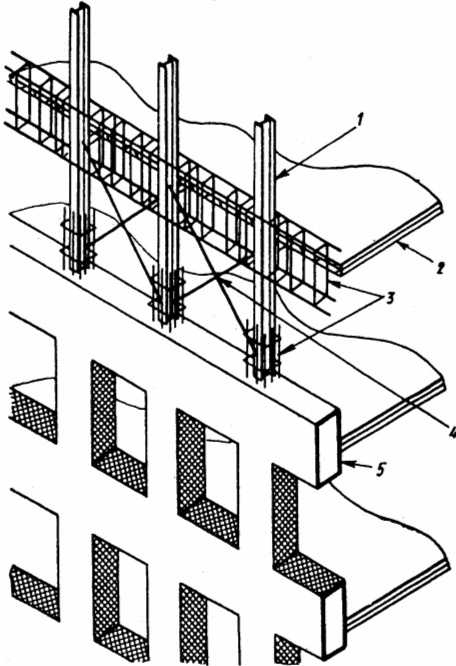
Hình IV.31. Sơ đồ nhà có kết cấu hộp liên hợp
