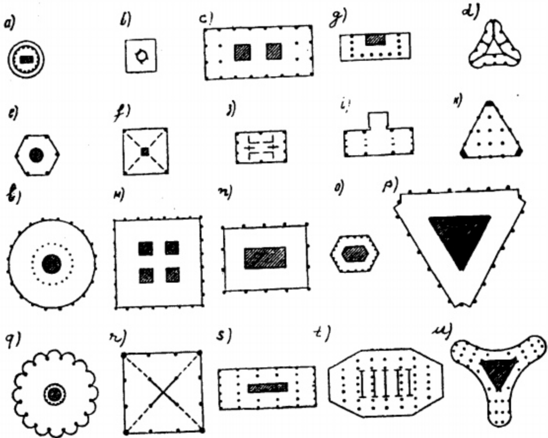
Hình IV.15. Nhà khung có lõi cứng
