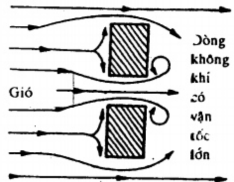
Gió Hình I.12
