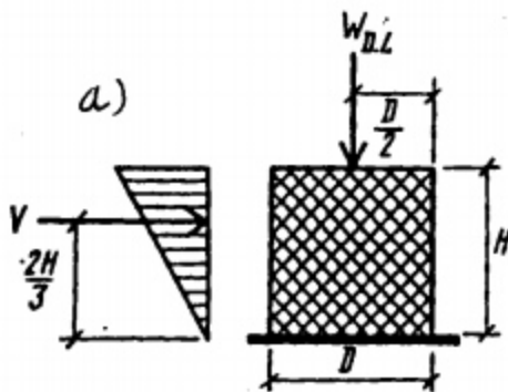
Hình I.25 a- Mặt cắt ;
