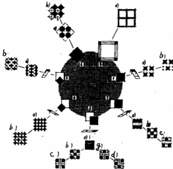
Hình VIII.8. Hệ cấu kiện môđun của cách ghép tấm với cột
