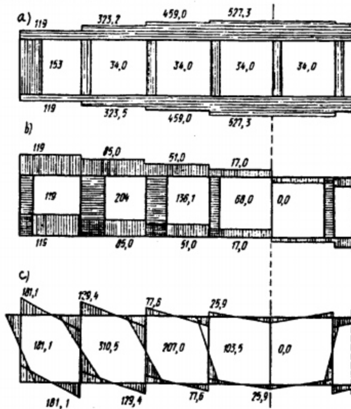
Hình VI.63 : Biểu đồ nội lực
