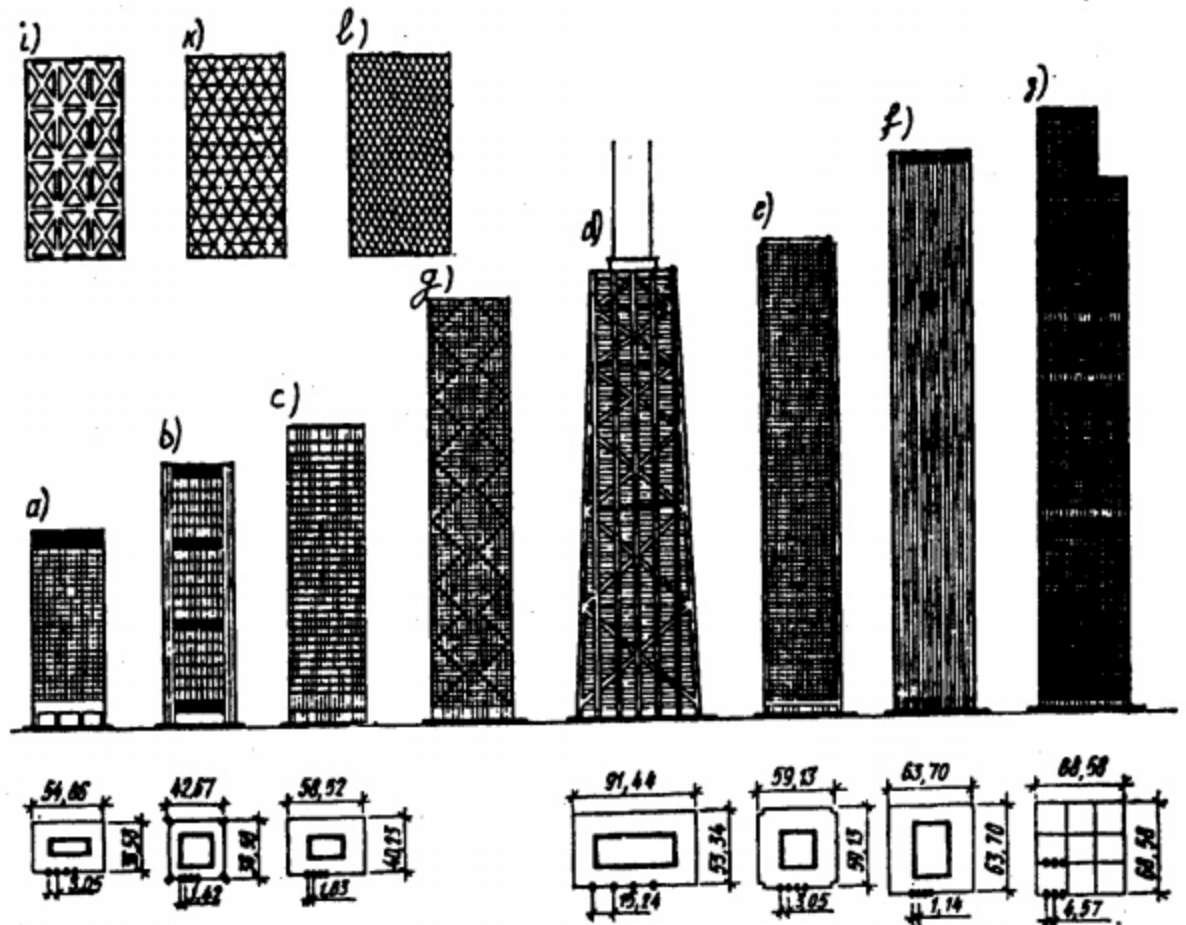
Hình IV.20. Kết cấu chịu lực của ngôi nhà dạng mạng lưới theo sơ đồ hộp
