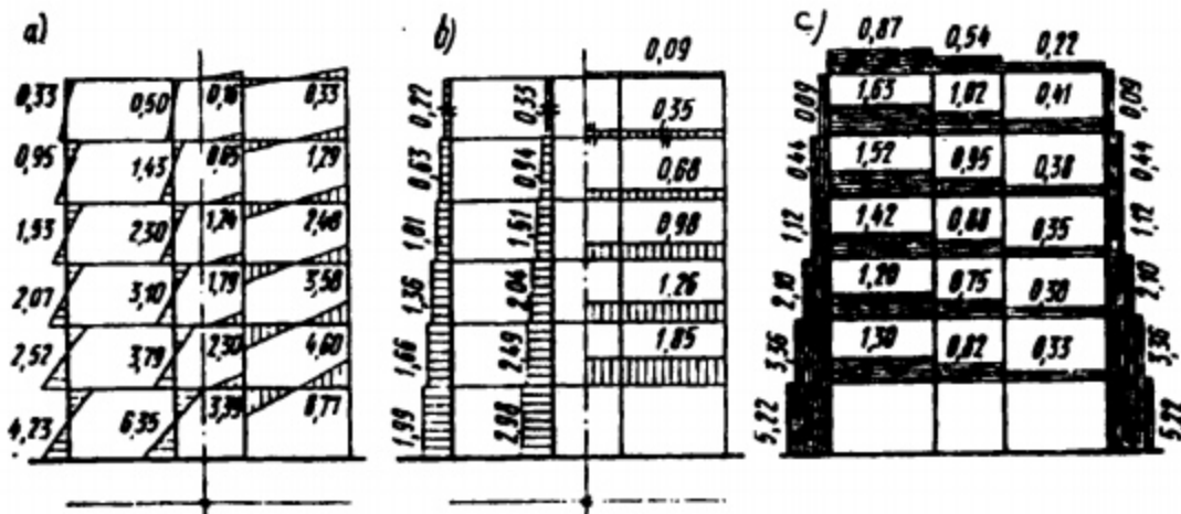
Hình VI.43 Biểu đồ nội lực a. Mômen uốn, Tm ; b - Lực dọc, T ; c - Lực dọc, T
