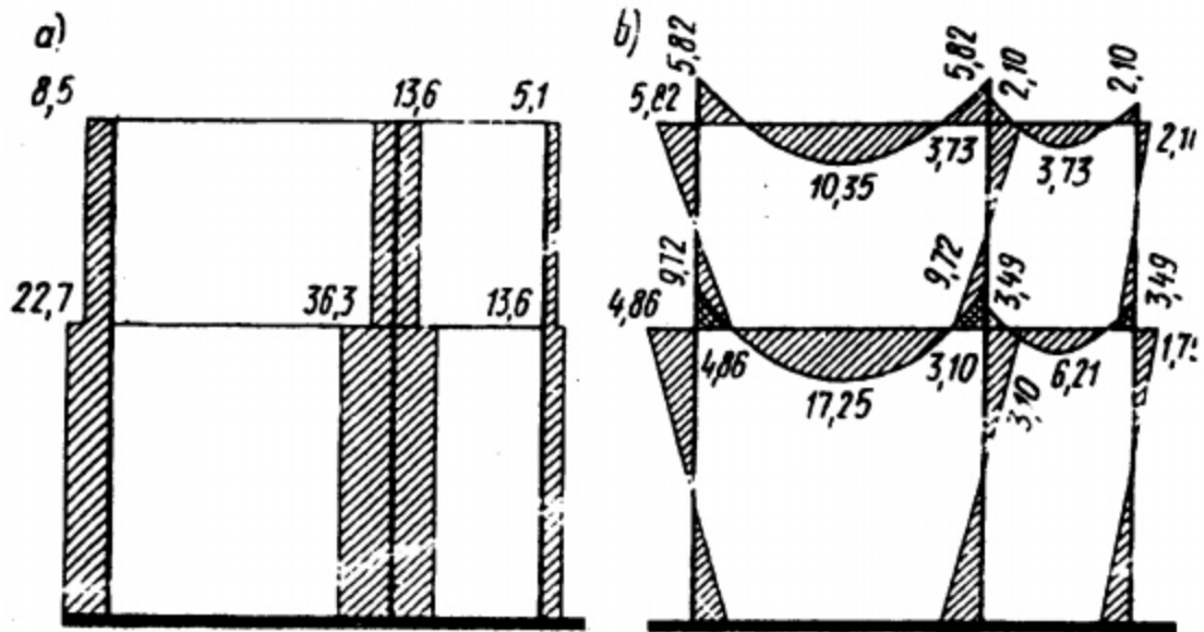
Hình VI-30. Biểu đồ nội lực a- Lực dọc, T ; b- Mômen uốn, M
