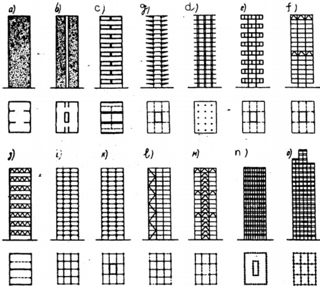
Hình II.1. Những sơ đồ kết cấu của nhà cao tầng
