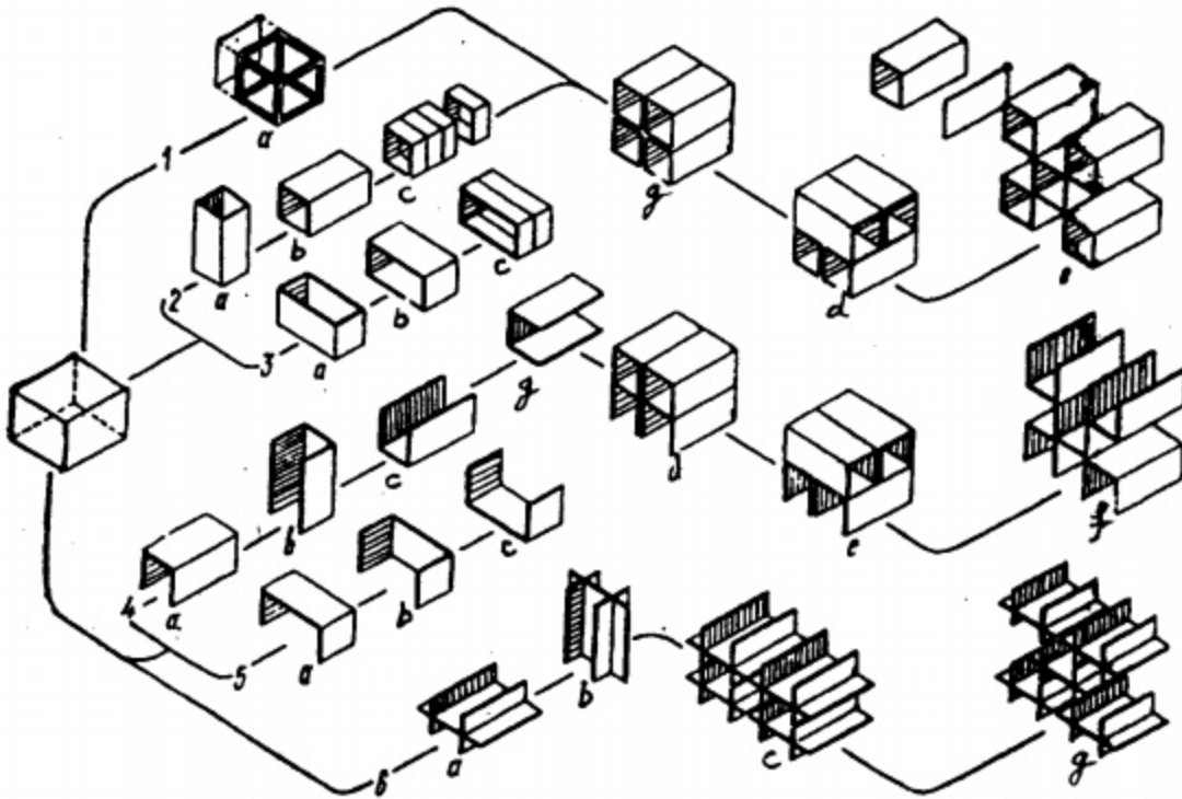
Hình VIII.10. Các bloc hình khối môđun chính
