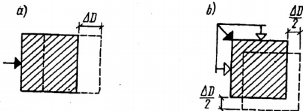
Hình I.9. Chuyển vị theo một trục (a), uốn theo 2 phương (b)
