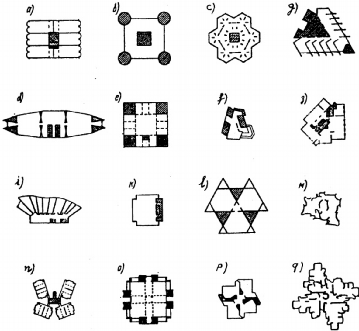
Hình IV.7. Nhà có tường và lõi cứng
