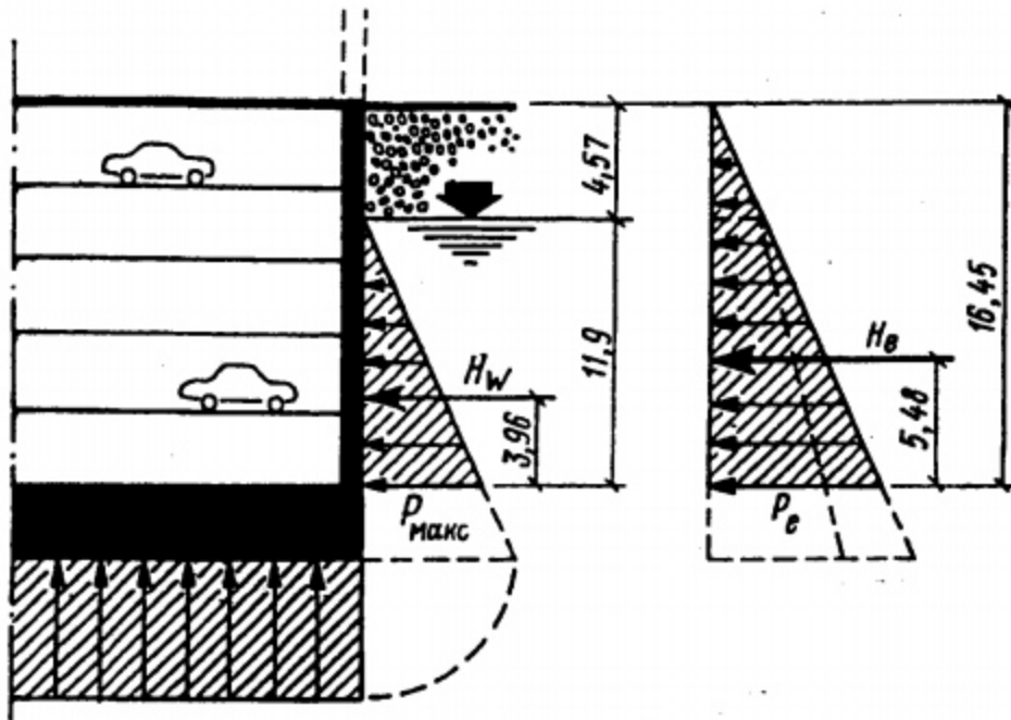
Hình 1.30. Áp lực bên của đất và nước tác dụng lên phần ngầm ngôi nhà
