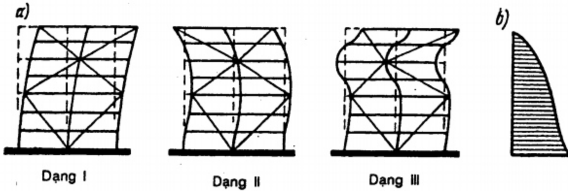
Hình 1.19- Các dạng dao động riêng của ngôi nhà (a) và biểu đồ lực cắt lớn nhất (b).
