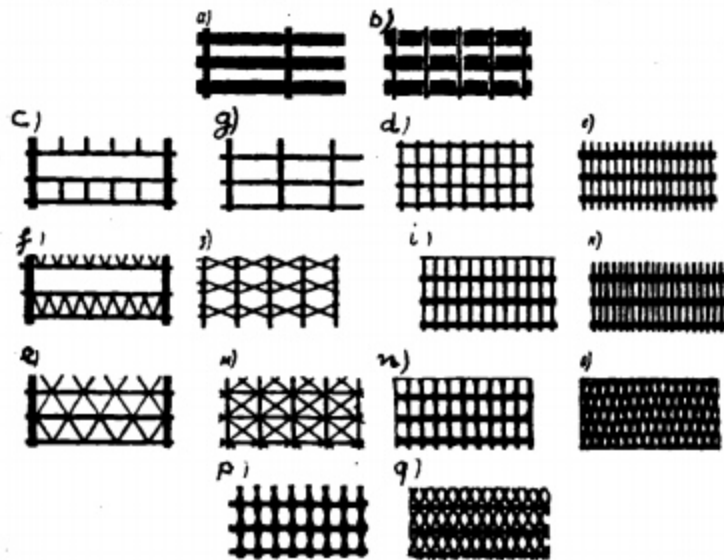
Hình III.11. Các kiểu kết cấu chịu lực dạng mạng lưới của tường ngoài
