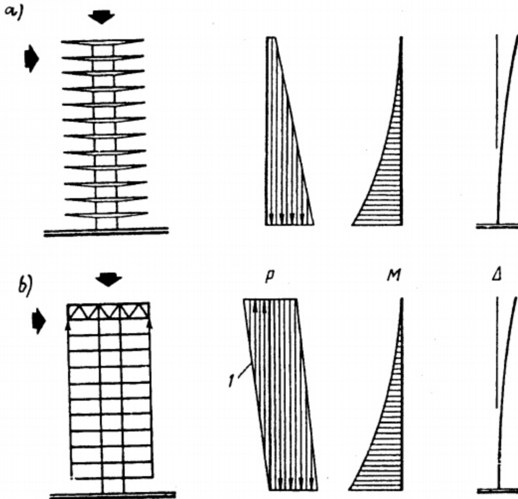
Hình IV.8. Nhà có các sàn công xôn (a) và nhà có các sàn treo (b)
