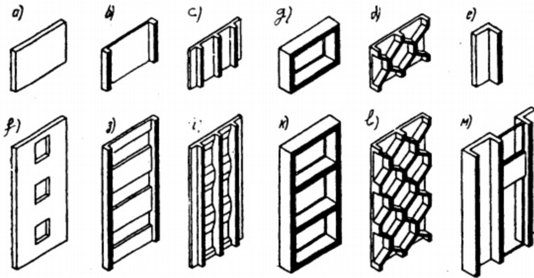
Hình VIII.7- Hệ panen tường chịu lực phía ngoài
