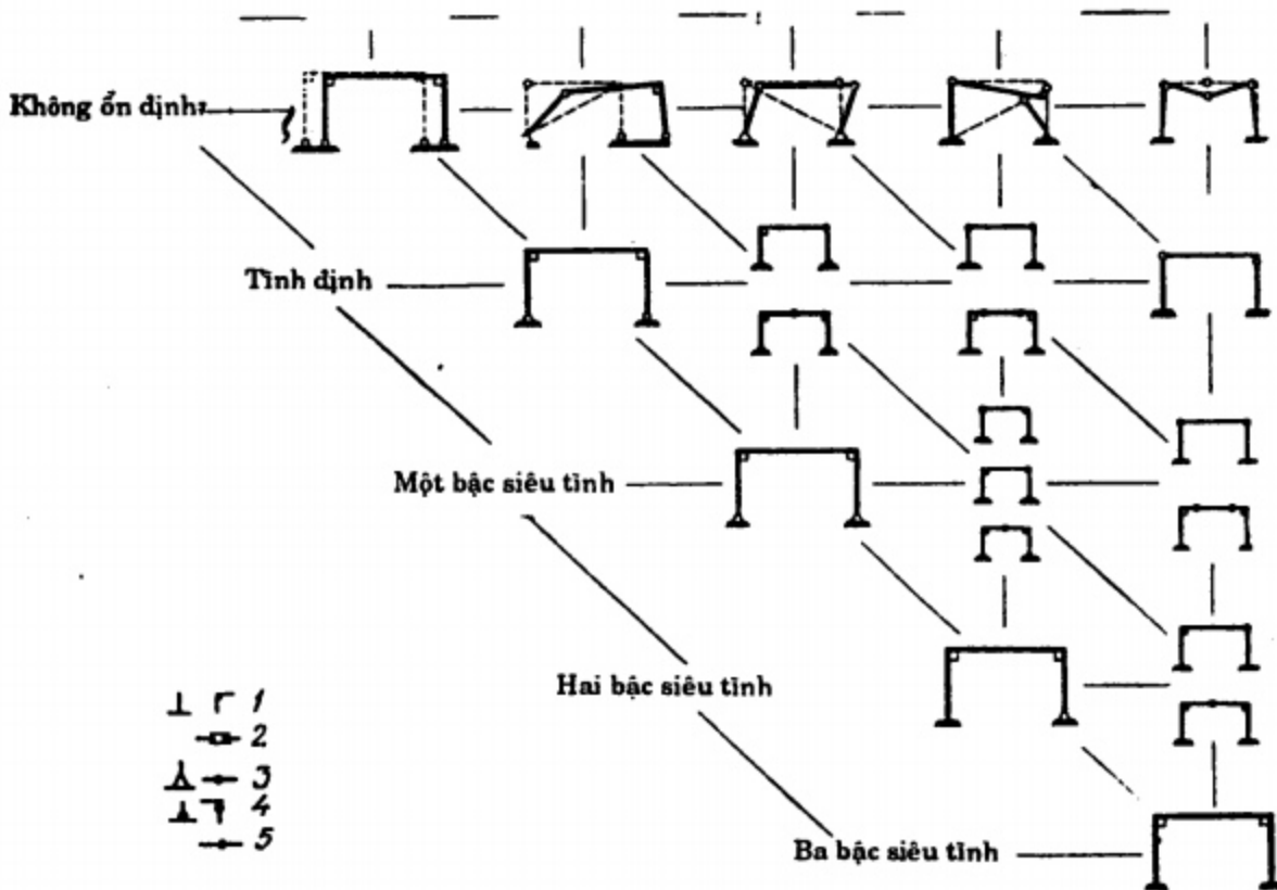
Hình VIII.2- Các dạng chính của khung chữ \Pi
