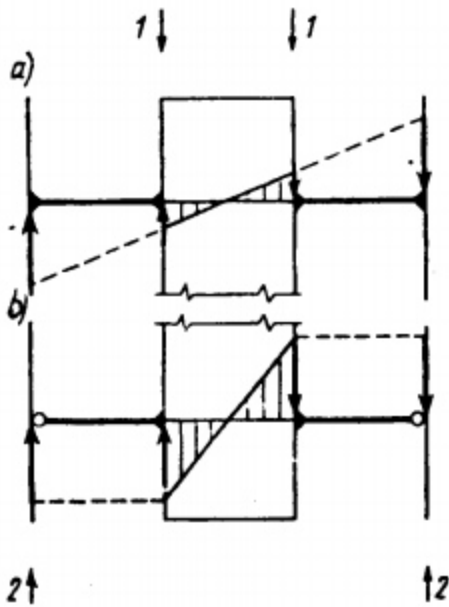
Hình IV.18. Biểu đồ ứng suất khi có các liên kết khác nhau
